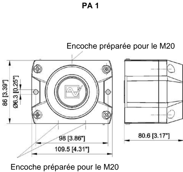
Schéma de perçage de l'intérieur du boîtier (PA 1)
