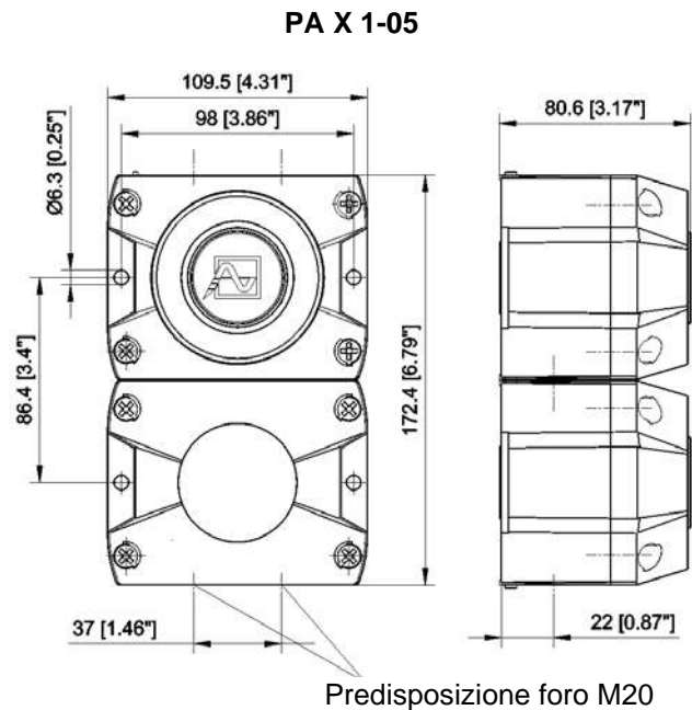
Schema forature interne all'alloggiamento (PA X 1-05)
