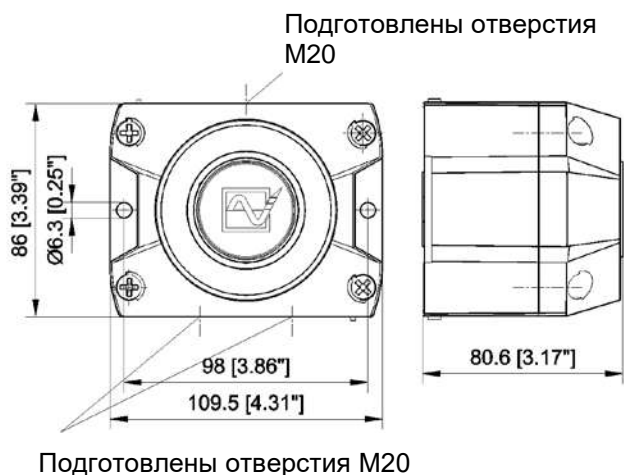
Схема расположения отверстий внутри корпуса (PA 1)
