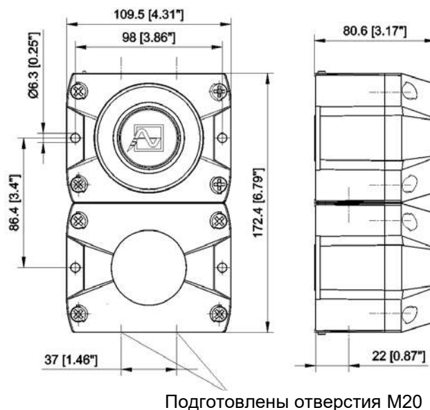
Схема расположения отверстий внутри корпуса (PA X 1-05)
