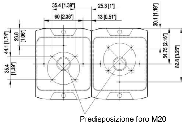
Schema forature interne all'alloggiamento (PA X 1-05)
