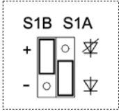
(auf der Treiberplatine)
